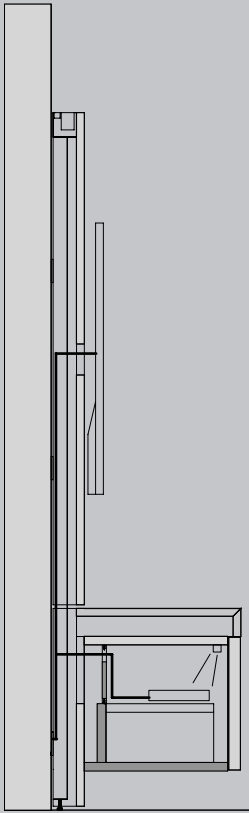
SOLUTION3 TV HANGING FROM PANELLING AND DECODER HOUSED INSIDE THE CONTAINER WITH FLAP DOOR - SIGNAL TRANSMITTED BY IR SOLUZIONE 3 TV APPESA A PANNELLATURA E DECODER ALLOGGIATO ALL'INTERNO DEL CONTENITORE CON ANTA A RIBALTA - TRASMISSIONE SEGNALE TRAMITE IR
