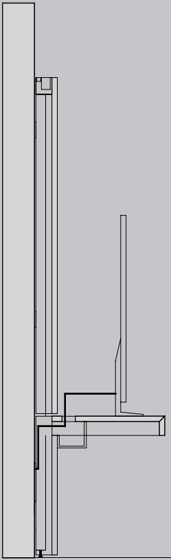
SOLUTION1 TV STANDING ON SUPPORT SHELF SOLUZIONE 1 TV APPOGGIATA A PIANO D'APPOGGIO SOLUTION2 TV HANGING FROM PANELLING AND DECODER STANDING ON SUPPORT SHELF SOLUZIONE 2 TV APPESA A PANNELLATURA E DECODER APPOGGIATO A PIANO D'APPOGGIO
